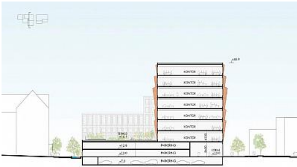
SEKTION B-B
